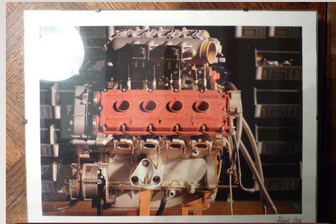
FERRARI MOTEUR
